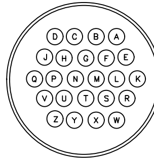
CHASSIS RECEPTACLE MS3102A-24-28S
