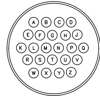
CABLE PLUG MS3106A-24-28P
